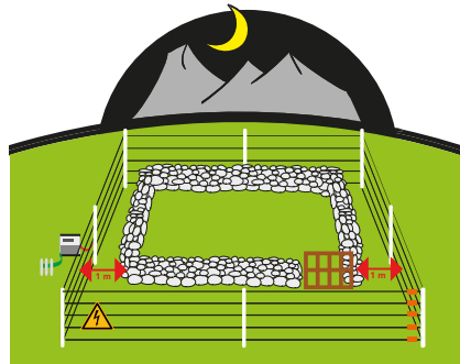
Zusätzliche Litzen
